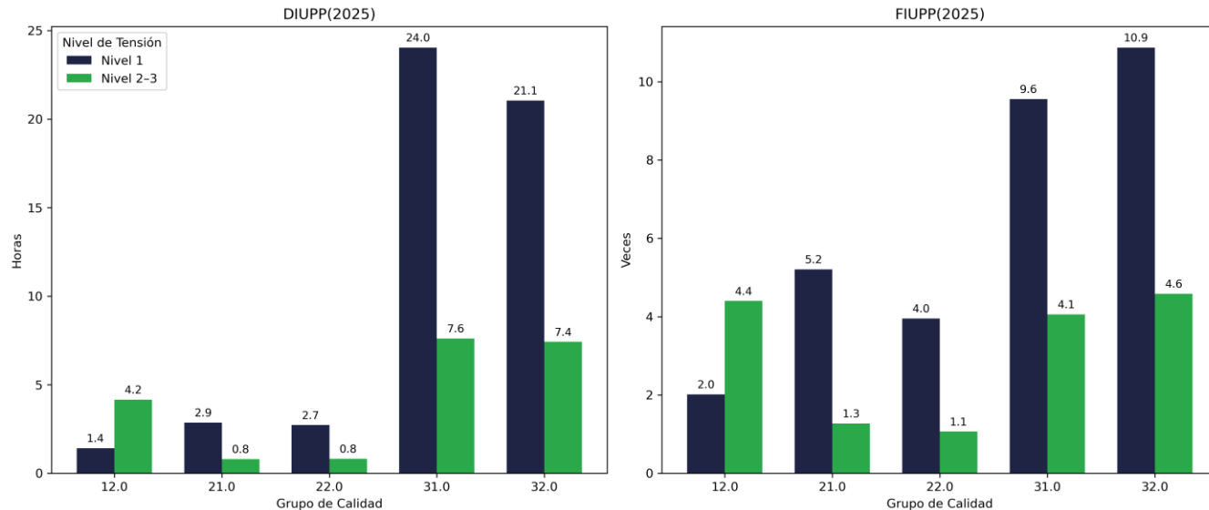
Figura 5. DIUPP y FIUPP por grupo de calidad y nivel de tensión - 2025 - EMPRESA DE ENERGIA DEL QUINDIO S.A.E.S.P.
