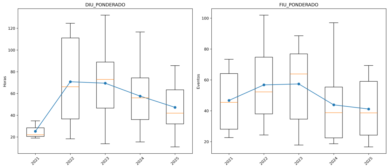
Figura 2. Evolución de los indicadores promedios ponderados DIU/FIU - ['EMPRESA DE ENERGIA DEL PUTUMAYO S.A. ESP']
