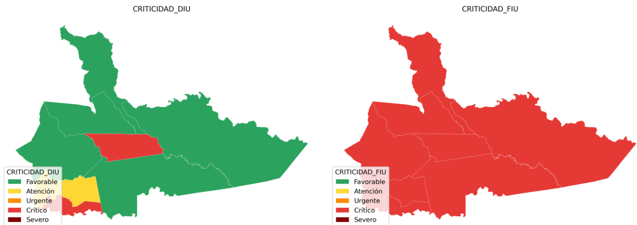
Figura 16. Mapa de grado criticidad de los indicadores DIU/FIU Promedio Ponderado por municipio - ['EMPRESA DE ENERGIA DEL PUTUMAYO S.A. ESP']
