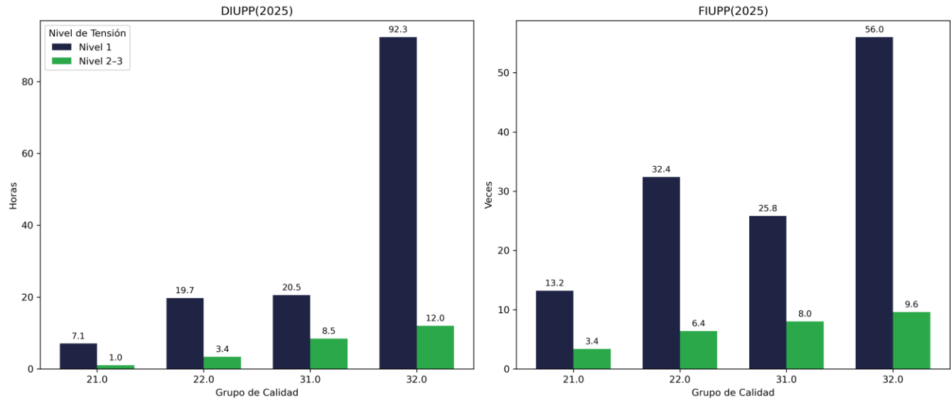
Figura 5. DIUPP y FIUPP por grupo de calidad y nivel de tensión - 2025 - EMPRESA DE ENERGIA DEL PUTUMAYO S.A. ESP
