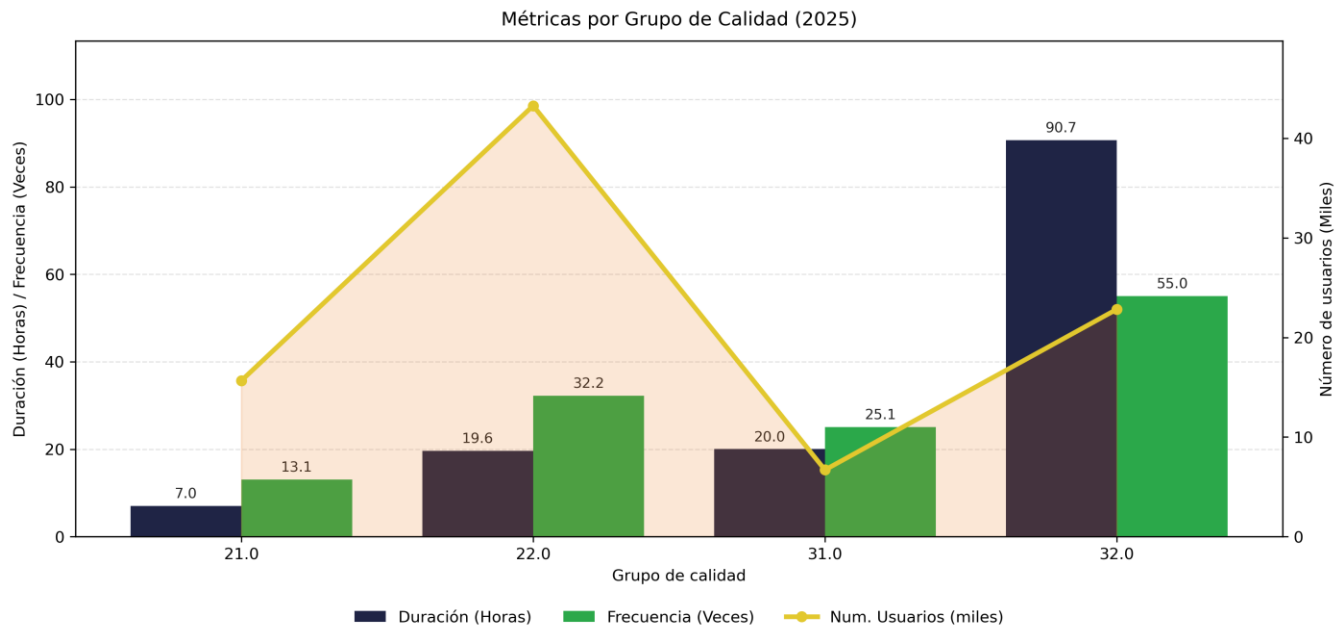
Figura 4. DIUPP y FIUPP por grupo de calidad - 2025 - EMPRESA DE ENERGIA DEL PUTUMAYO S.A. ESP
