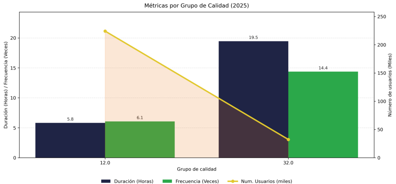
Figura 4. DIUPP y FIUPP por grupo de calidad - 2025 - EMPRESA DE ENERGÍA DE PEREIRA S.A. ESP.
