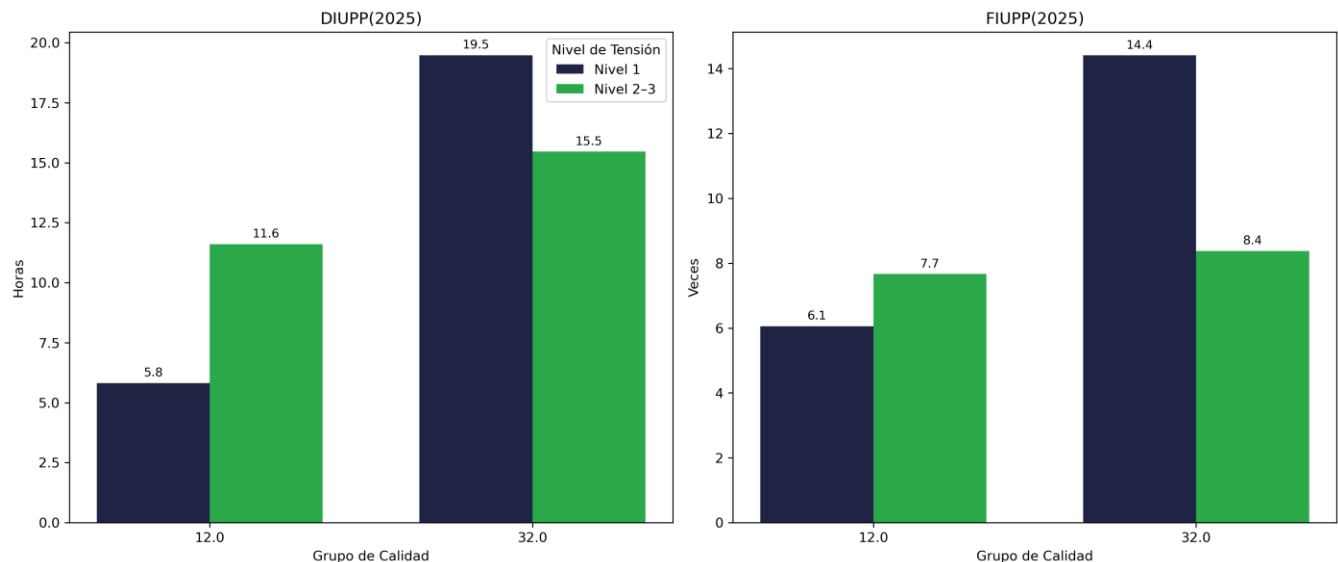
Figura 5. DIUPP y FIUPP por grupo de calidad y nivel de tensión - 2025 - EMPRESA DE ENERGÍA DE PEREIRA S.A. ESP.
