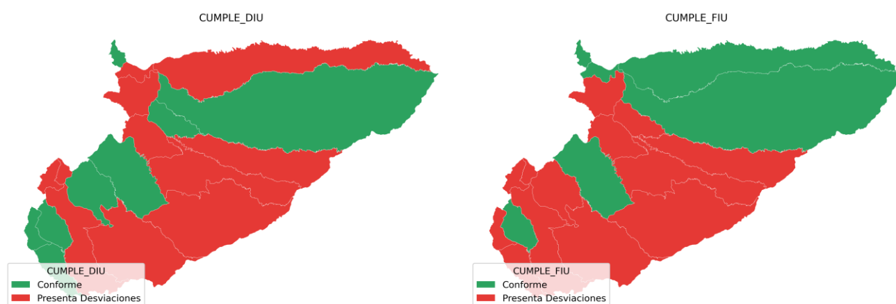
Figura 6. Mapa de conformidad con los indicadores DIU/FIU Promedio Ponderado por municipio - [EMPRESA DE ENERGIA DE CASANARE SA ESP]
