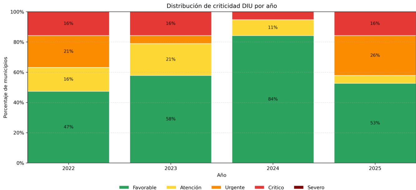
Figura 19. Distribución de criticidad DIUPP por año - EMPRESA DE ENERGIA DE CASANARE
