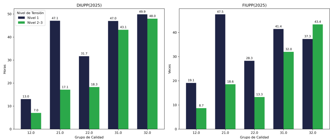
Figura 5. DIUPP y FIUPP por grupo de calidad y nivel de tensión - 2025 - EMPRESA DE ENERGIA DE CASANARE
