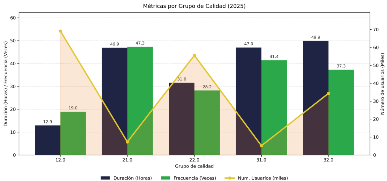
Figura 4. DIUPP y FIUPP por grupo de calidad - 2025 - EMPRESA DE ENERGIA DE CASANARE
