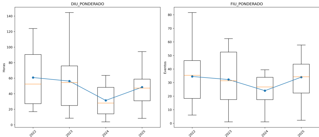
Figura 2. Evolución de los indicadores promedios ponderados DIU/FIU - ['EMPRESA DE ENERGIA DE CASANARE SA ESP']
