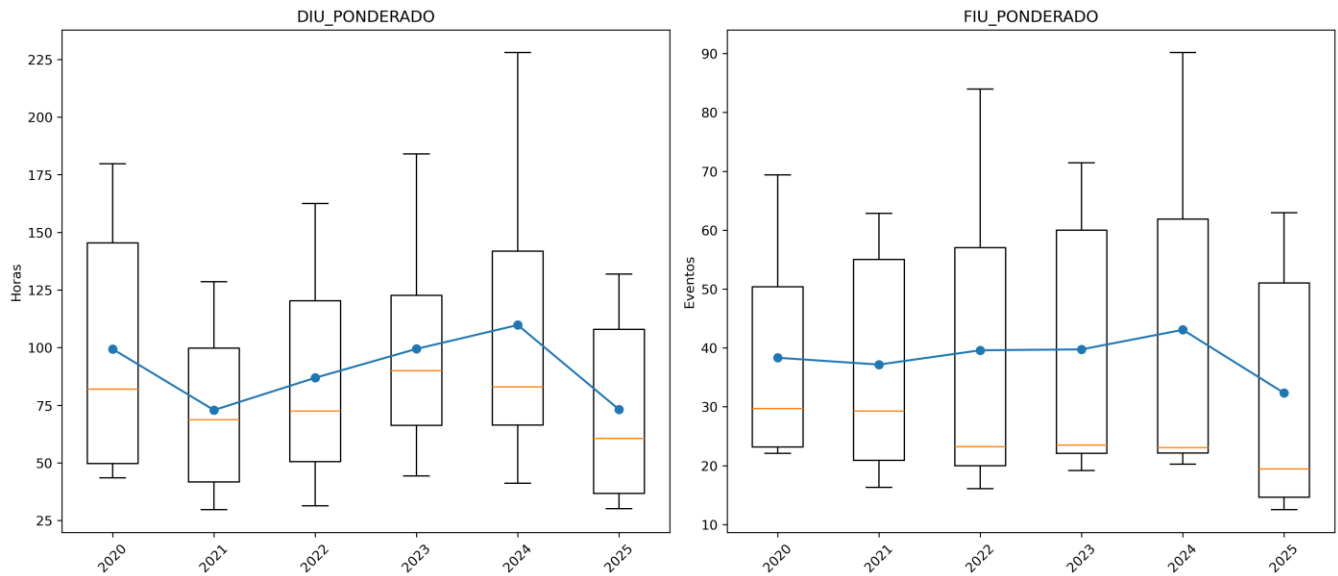
Figura 2. Evolución de los indicadores promedios ponderados DIU/FIU - ['EMPRESA DE ENERGIA DE ARAUCA']
