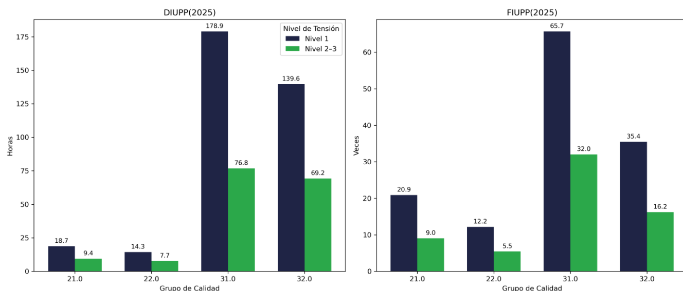
Figura 5. DIUPP y FIUPP por grupo de calidad y nivel de tensión - 2025 - EMPRESA DE ENERGIA DE ARAUCA
