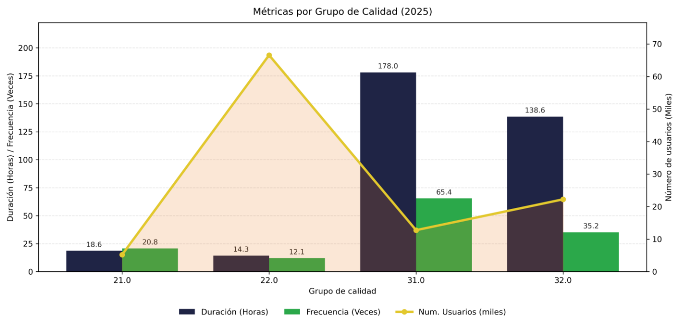
Figura 4. DIUPP y FIUPP por grupo de calidad - 2025 - EMPRESA DE ENERGIA DE ARAUCA
