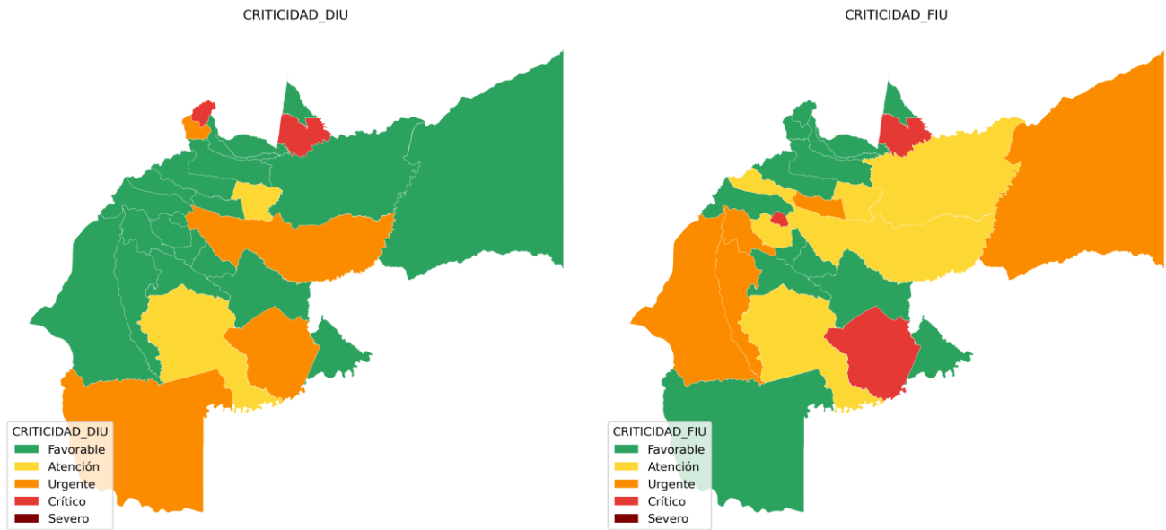
Figura 22. Mapa de grado criticidad de los indicadores DIU/FIU Promedio Ponderado por municipio - ['ELECTRIFICADORA DEL META S.A. E.S.P.']
