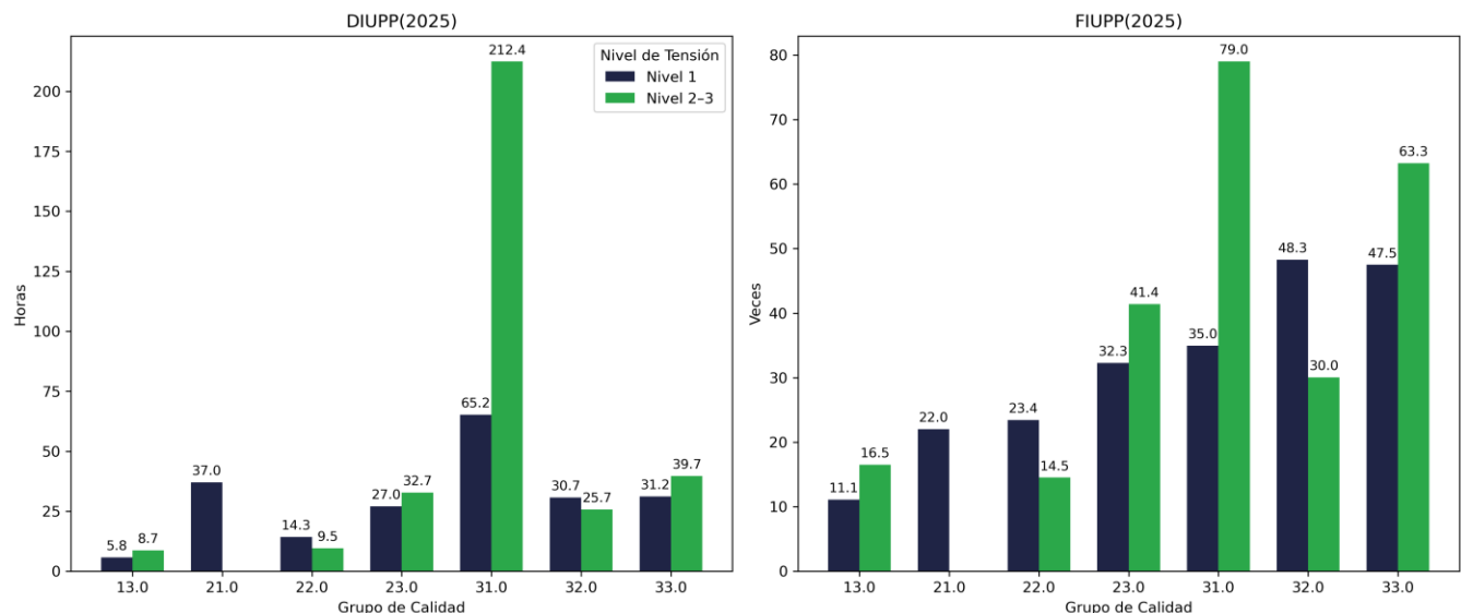
Figura 5. DIUPP y FIUPP por grupo de calidad y nivel de tensión - 2025 - ELECTRICADORA DEL META S.A. E.S.P.
