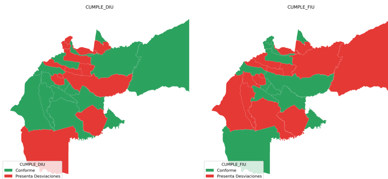
Figura 6. Mapa de conformidad con los indicadores DIU/FIU Promedio Ponderado por municipio - [ELECTRIFICADORA DEL META S.A. E.S.P.]
