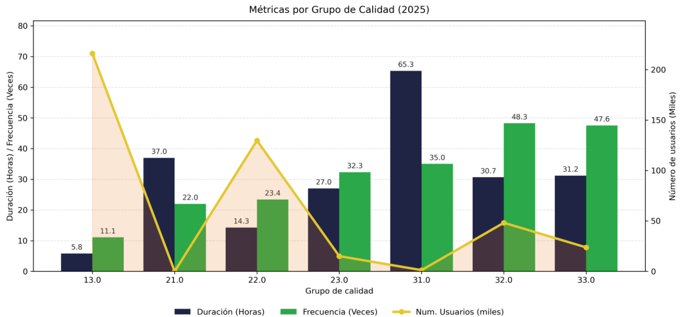
Figura 4. DIUPP y FIUPP por grupo de calidad - 2025 - ELECTRICADORA DEL META S.A. E.S.P.
