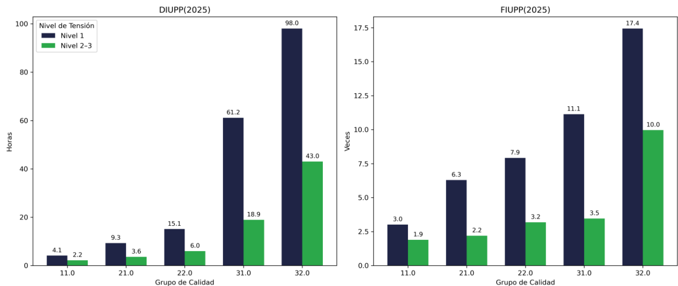
Figura 5. DIUPP y FIUPP por grupo de calidad y nivel de tensión - 2025 - ELECTRICADORA DEL HUILA S.A. E.S.P.
