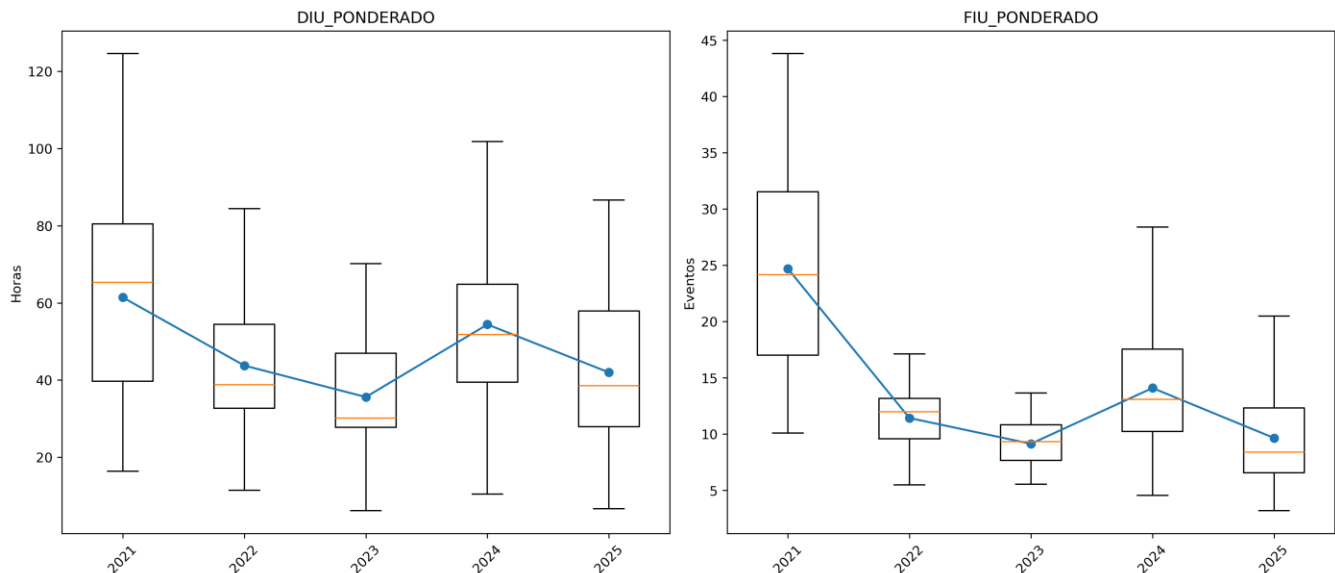
Figura 2. Evolución de los indicadores promedios ponderados DIU/FIU - ['ELECTRIFICADORA DEL HUILA S.A. E.S.P.']
