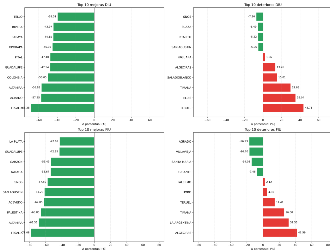
Figura 3. Municipios con mayores mejoras y deterioros DIUPP/FIUPP - ['ELECTRIFICADORA DEL HUILA S.A. E.S.P.']
