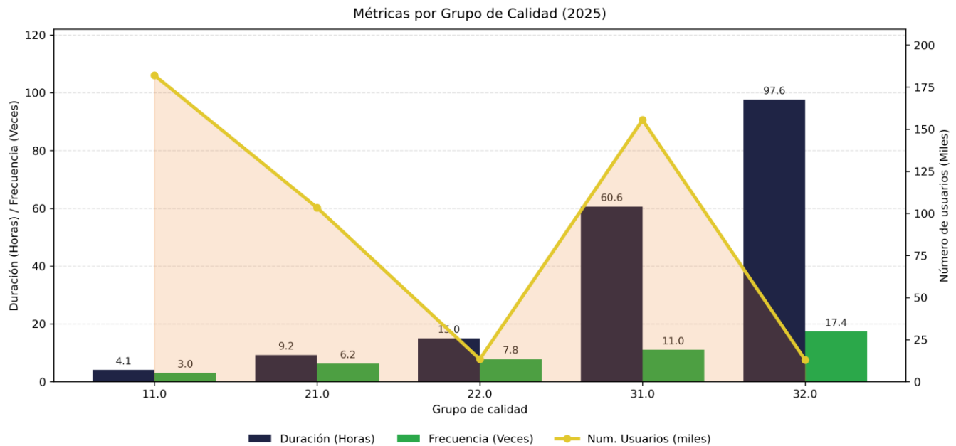
Figura 4. DIUPP y FIUPP por grupo de calidad - 2025 - ELECTRICADORA DEL HUILA S.A. E.S.P.
