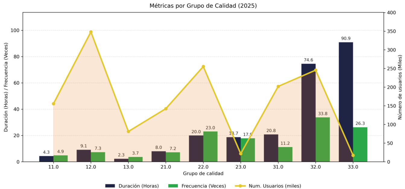
Figura 4. DIUPP y FIUPP por grupo de calidad - 2025 - CELSIA COLOMBIA S.A.S. E.S.P.
