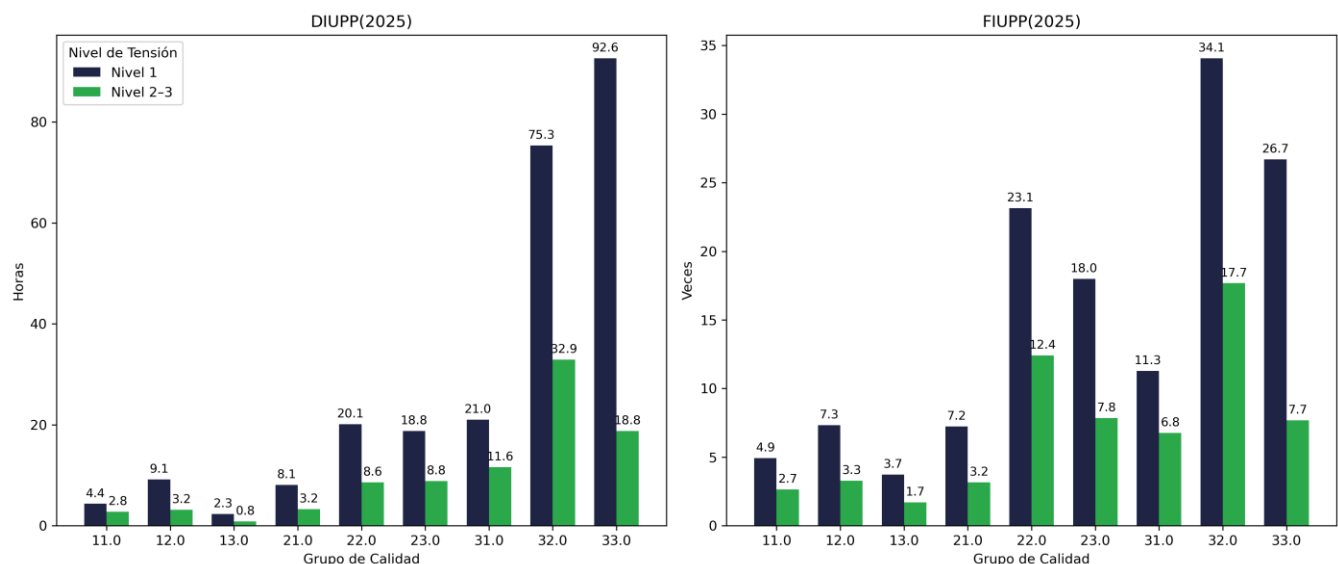
Figura 5. DIUPP y FIUPP por grupo de calidad y nivel de tensión - 2025 - CELSIA COLOMBIA S.A.S. E.S.P.
