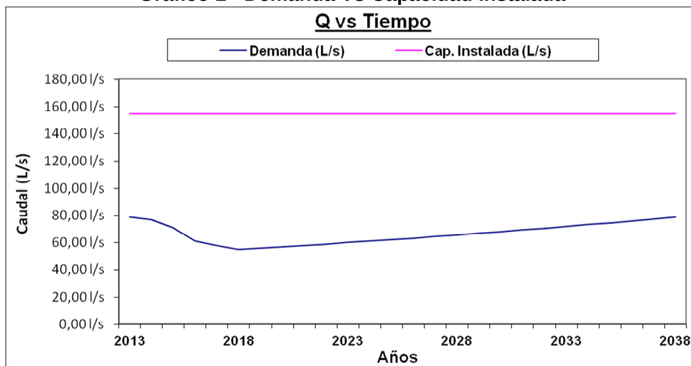
Gráfico 1 - Demanda Vs Capacidad Instalada
