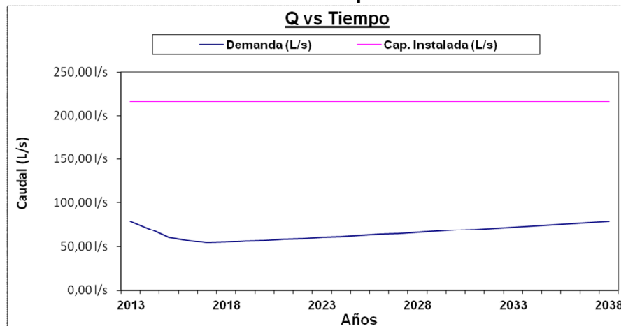
Gráfico 2 - Demanda Vs Capacidad Instalada
