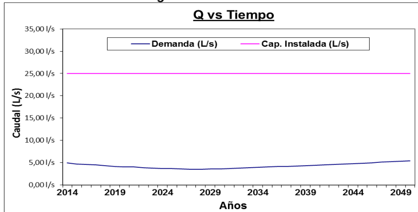
Imagen 3. Balance Hidráulico
