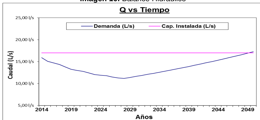
Imagen 10. Balance Hidráulico
