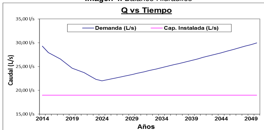
Imagen 4. Balance Hidráulico
