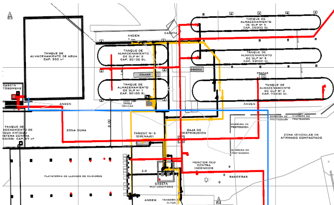
GRAFICA 3.1. DISPOSICION PLANTA DE ALMACENAMIENTO DE GLP EN PEREIRA.
