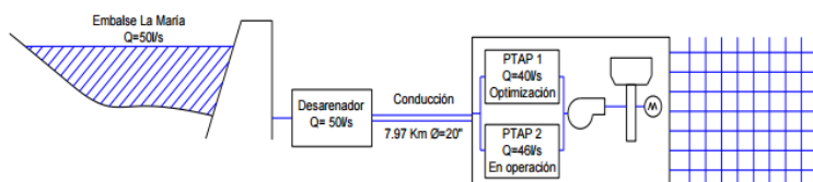
Ilustración 1 Esquema estructural servicio de acueducto
