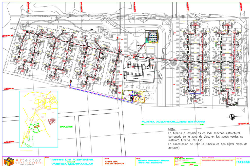
Imagen 23. Diagrama del sistema de alcantarillado público Ciudadela del Viento y Torres de Alamadina
