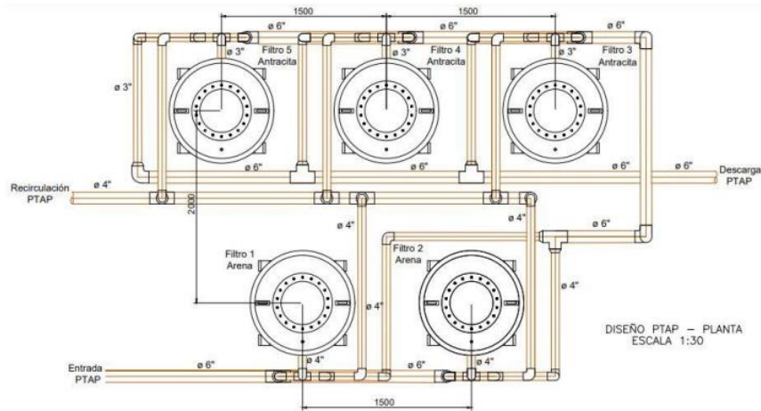
Imagen 9. Vista en planta PTAP
